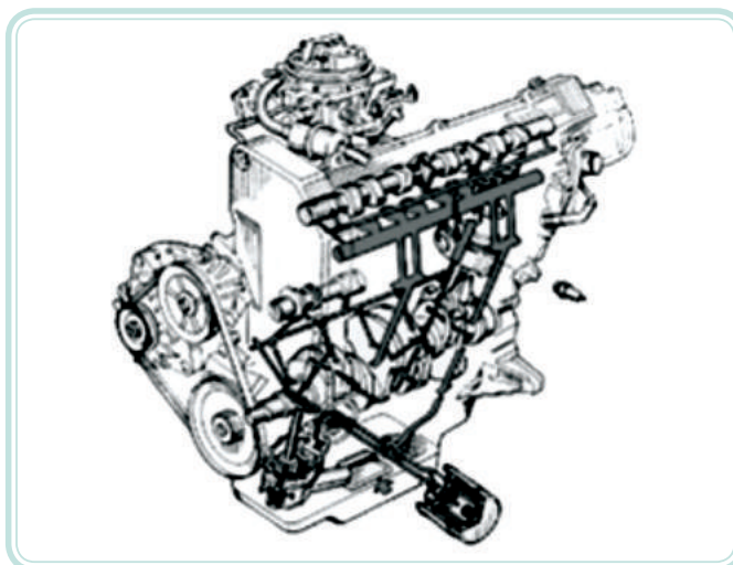
Figura 4.49: Galerias do óleo lubrificante
