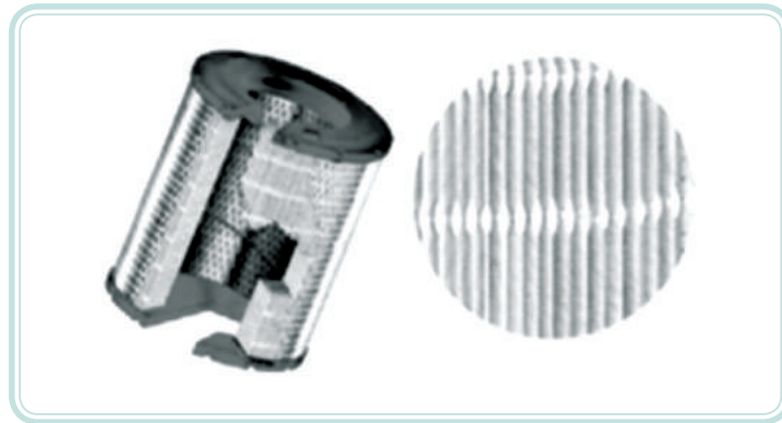
Figura 4.3: Elemento primário
