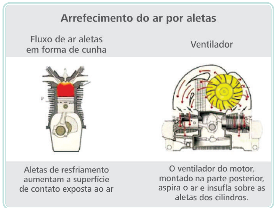
Figura 4.36: Refrigeração a ar nos motores
