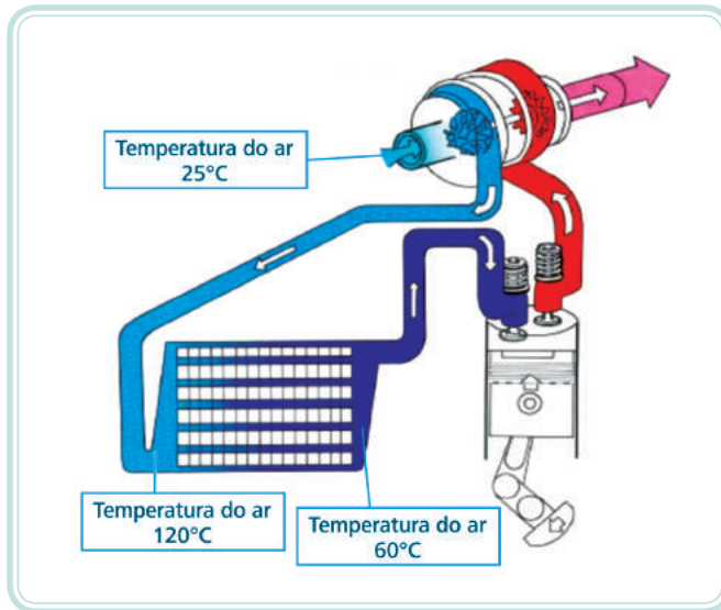
Figura 4.12: Esquema de funcionamento do resfriamento do ar Fonte: CTISM, adaptado de Mercedes Benz do Brasil, 2006
