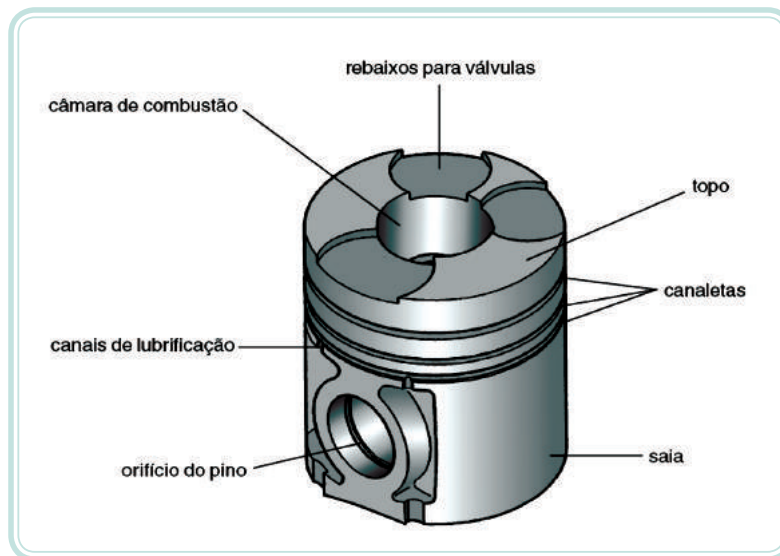
Figura 2.14: Denominação das partes constituintes de um pistão
