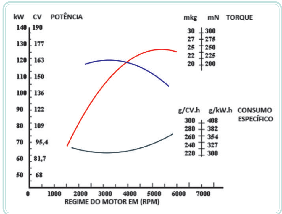
Figura 8.1: Curvas características da avaliação de desempenho
