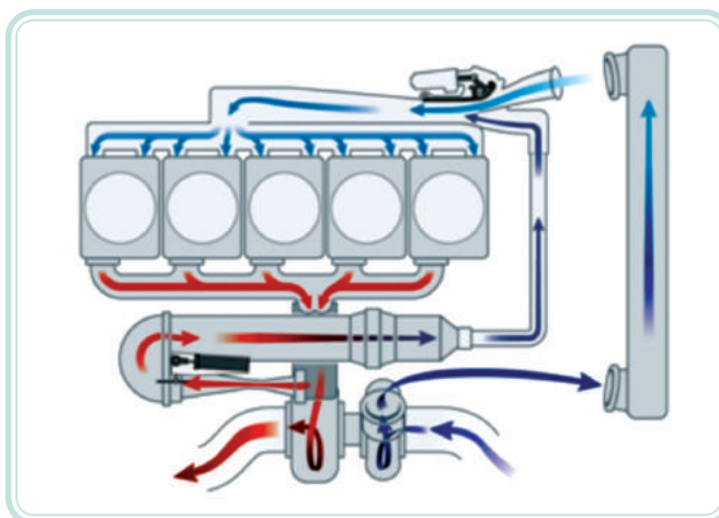
Figura 4.13: Esquema de circulação do ar no motor Fonte: Mercedes Benz do Brasil, 2006
