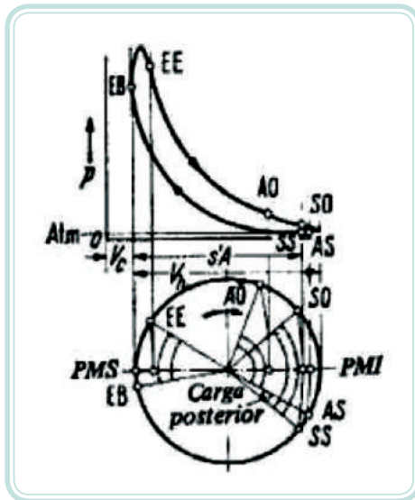
Figura 6.12: Gráfico de pressões em um motor ciclo Diesel de dois tempos com válvula de admissão no cabeçote e fendas de exaustão por fluxo contínuo
