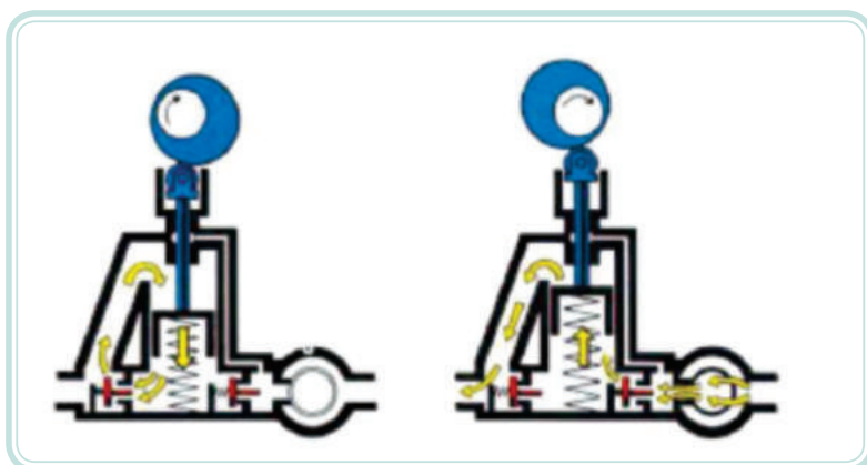
Figura 4.18: Esquema de funcionamento da bomba de alimentação de combustível
